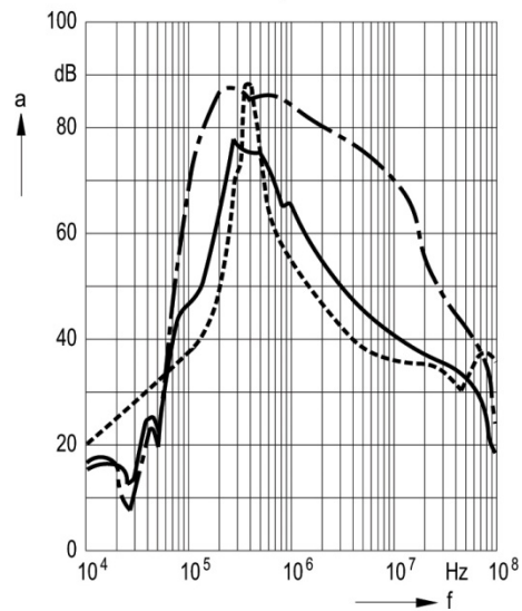
KRF1600VCB, KRF2500VCB
