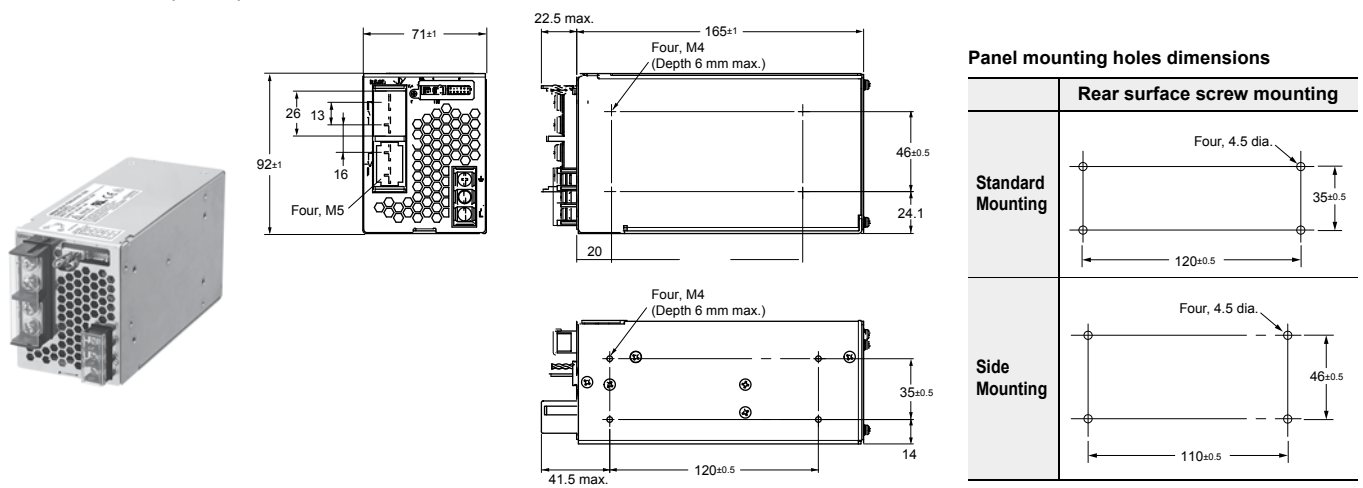
S8JX-P300□□N (300 W)
