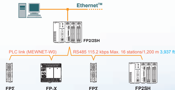
FP2-MCU (AFP2465)
