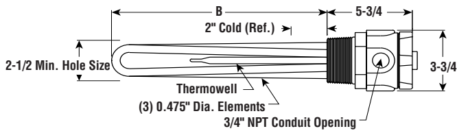
E2 — Dimensions (Inches)
