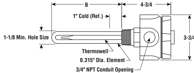
E2 — Dimensions (Inches)
