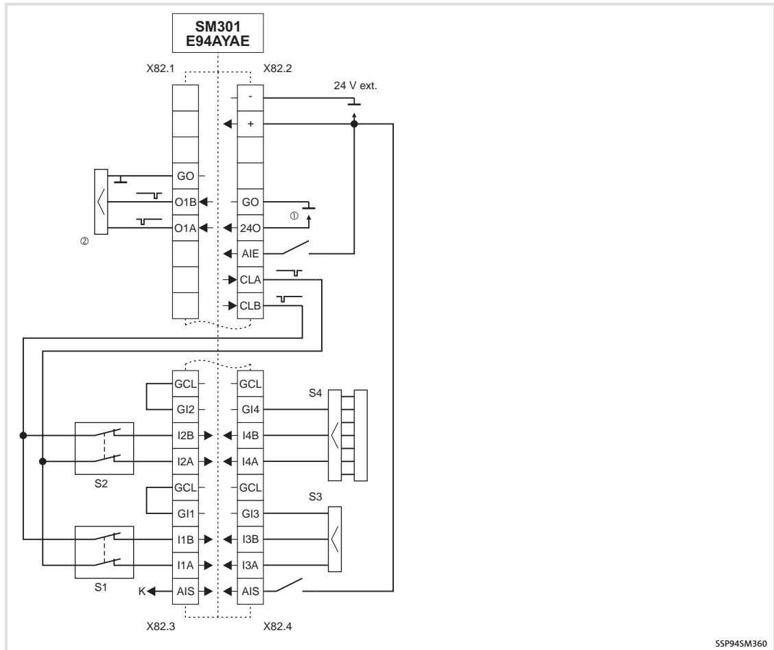
Fig. 1-3 Wiring example
