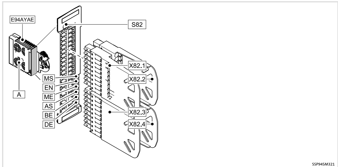
Fig. 1-2 Module view
