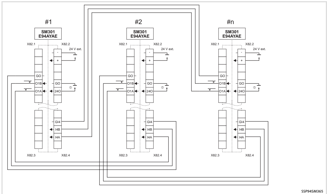
Fig. 1-11 Wiring example
