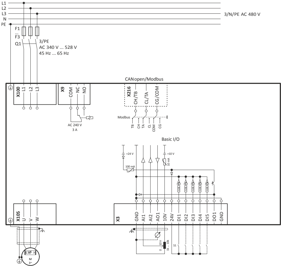
Fig. 3: Wiring example
