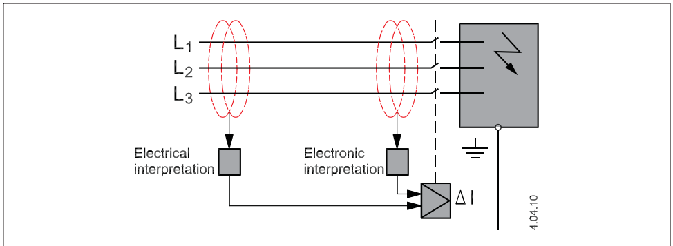
Fig. 6.8 Universal RCCB
