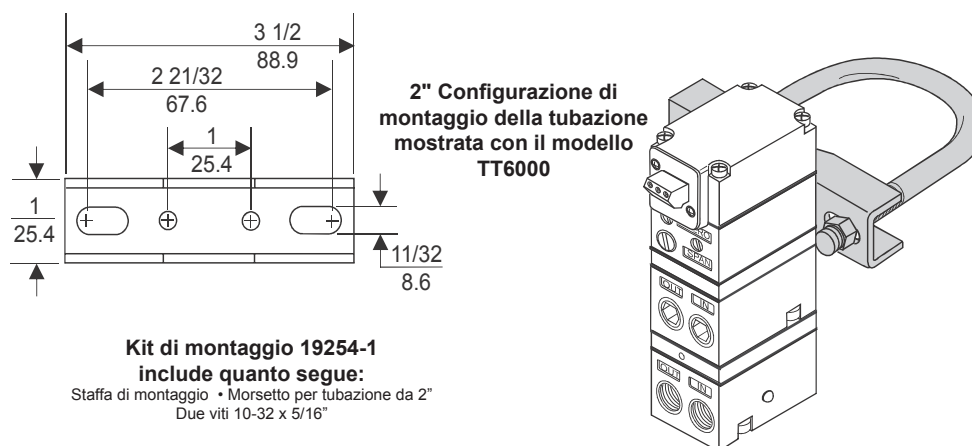
Figura 8. Kit di montaggio 19254-1 (venduto separatamente)
