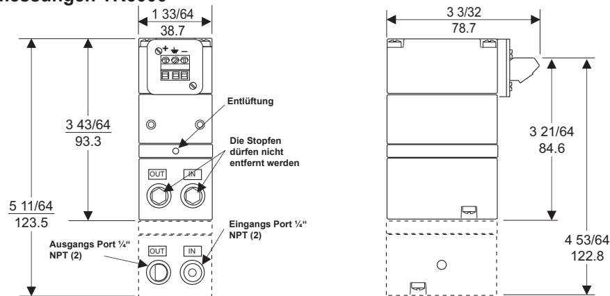
Abbildung 4. Außenabmessungen TR6000
