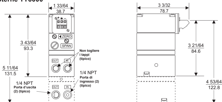
Figura 2. Dimensioni esterne TT6000
