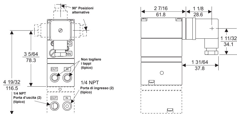
Figura 3. Dimensioni esterne TD6000
