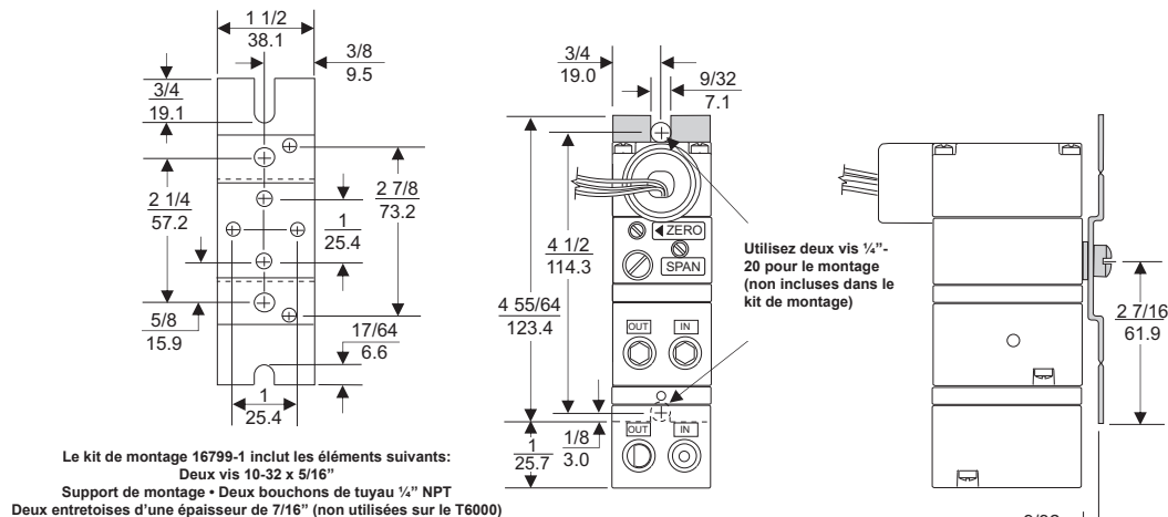
Figure 6. Kit de montage 16799-1 (Inclus avec l'unité)
