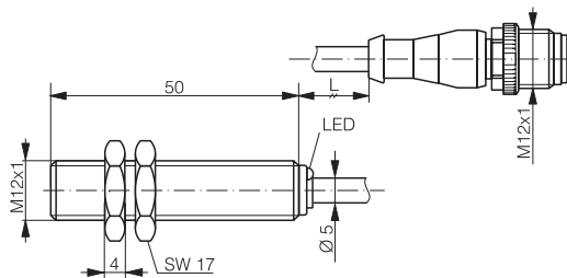
DW-AV-70#-M12-274
