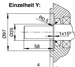
Einzelheit Y:
