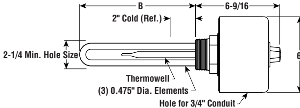
E1 — Dimensions (Inches)
